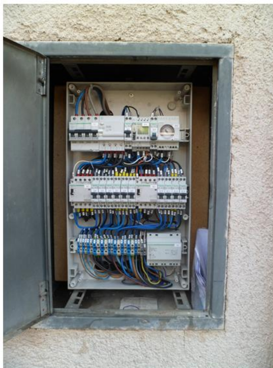
Fig. 9 – Il quadro installato a Varollo
