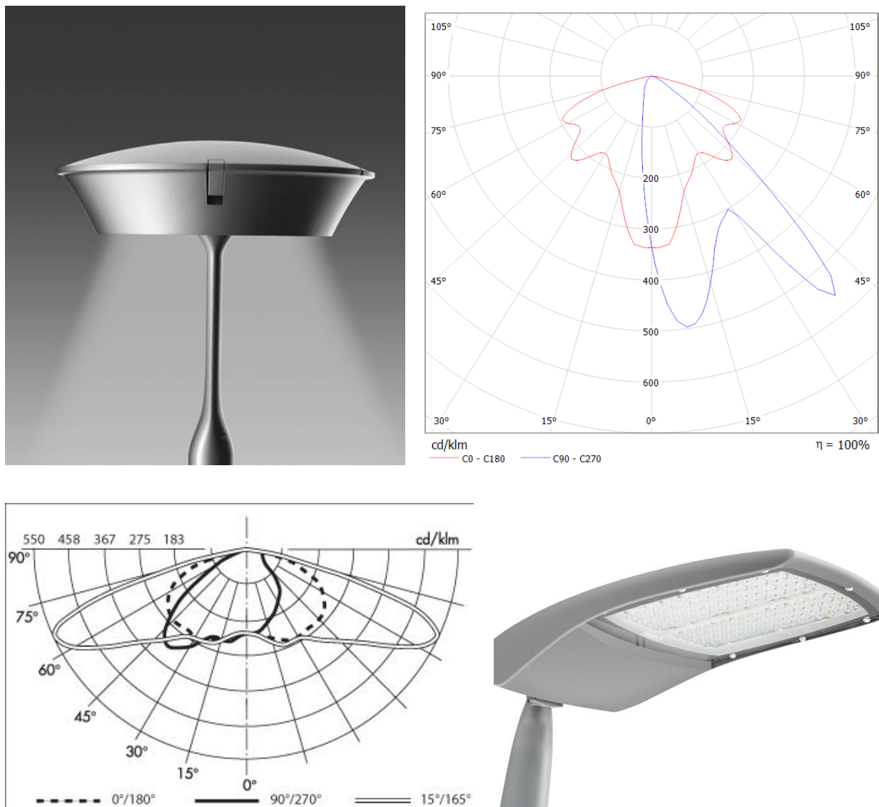
Fig. 24 – Esempi di corpo illuminante a LED con relativa curva fotometrica utilizzabile per le nuove installazioni o sostituzioni
