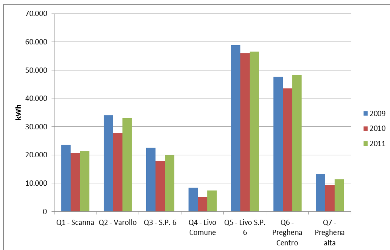
Grafico 3 – Ripartizione per quadro elettrico dei consumi relativi al triennio 2009-2011 - Livo
