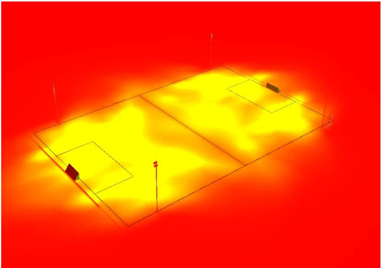
Fig. 27 - Campo sportivo di Rumo - Rendering a colori sfalsati frutto della simulazione con apposito software illuminotecnico
