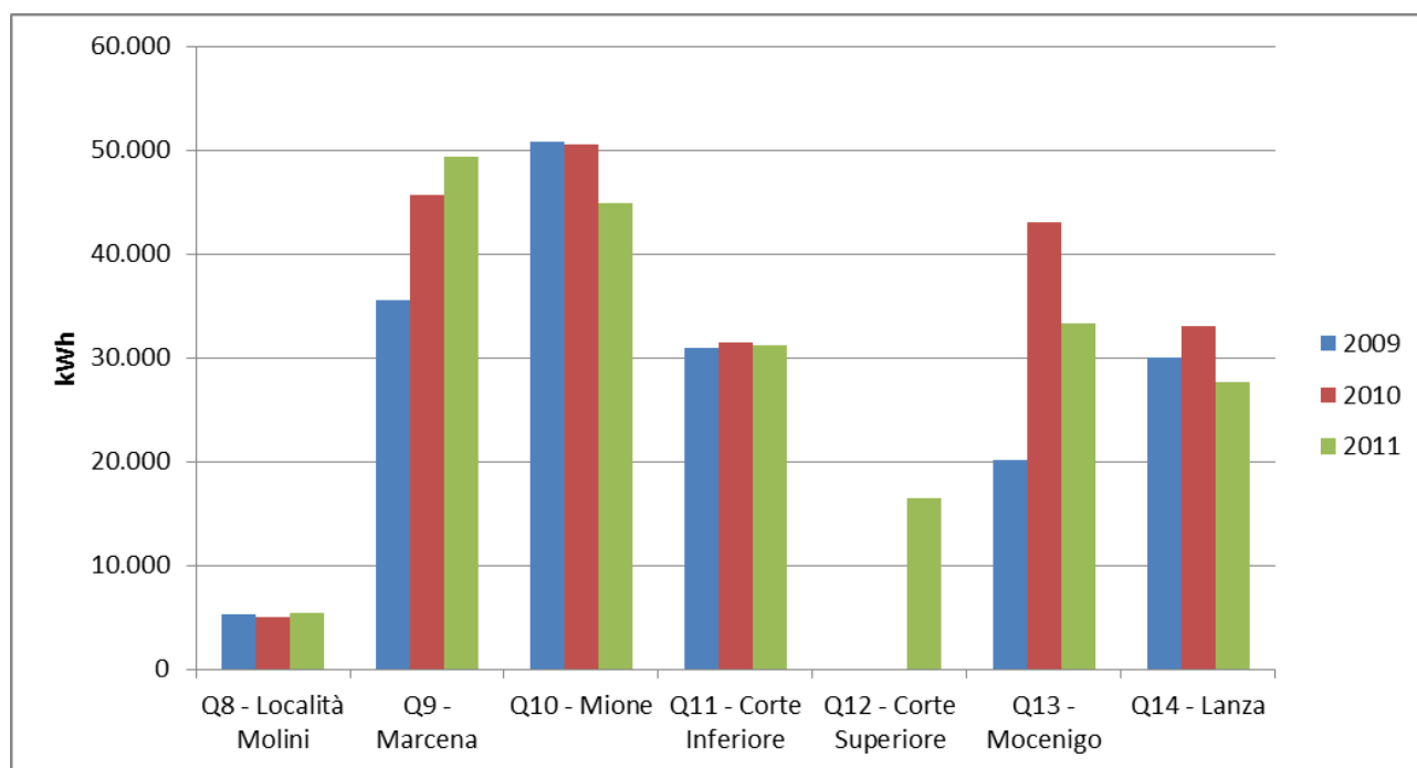
Grafico 4 - Ripartizione per quadro elettrico dei consumi relativi al triennio 2009-2011 - Rumo
