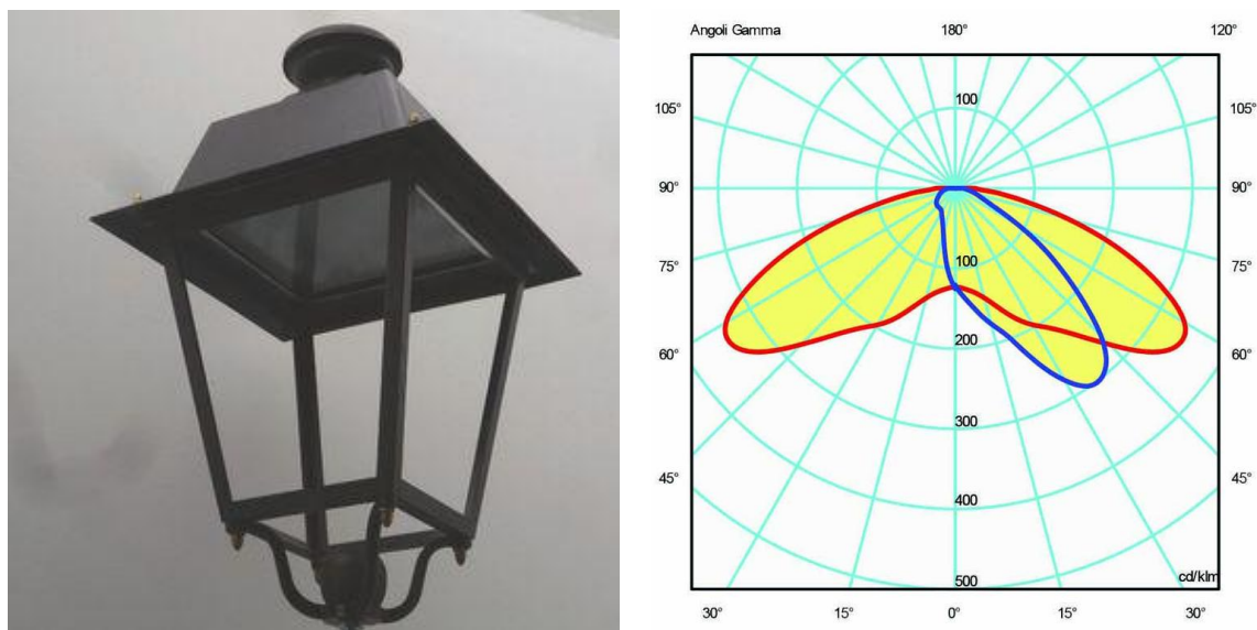
Fig. 23 – Corpo illuminante a LED da arredo urbano, proposto in alcuni tratti e relativa curva fotometrica.
