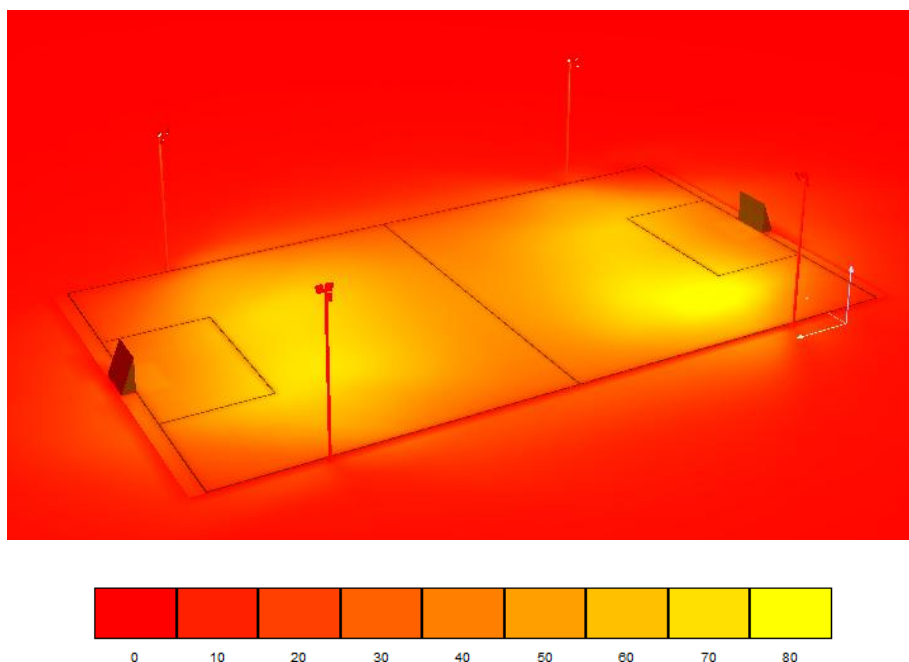
Fig. 26 – Rendering a colori sfalsati del campo da gioco di Livo
